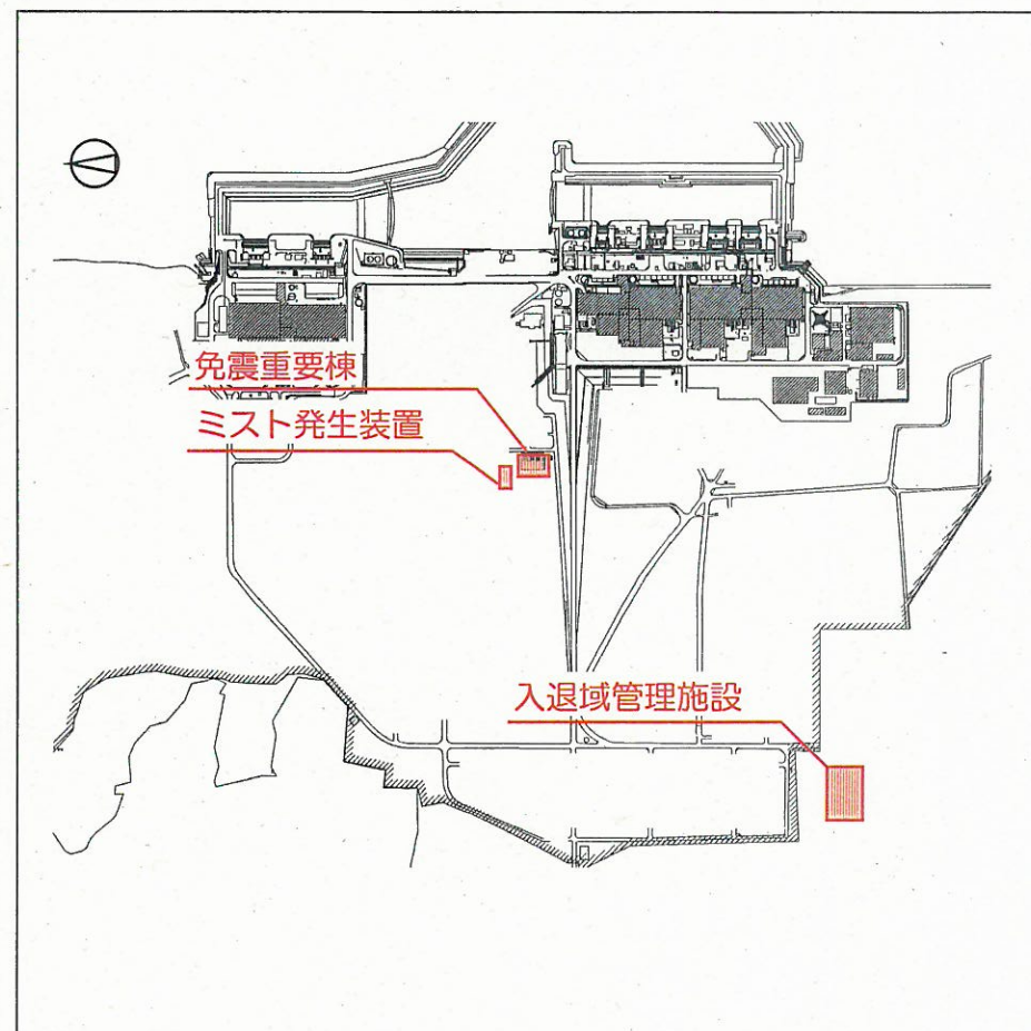
構内配置図
