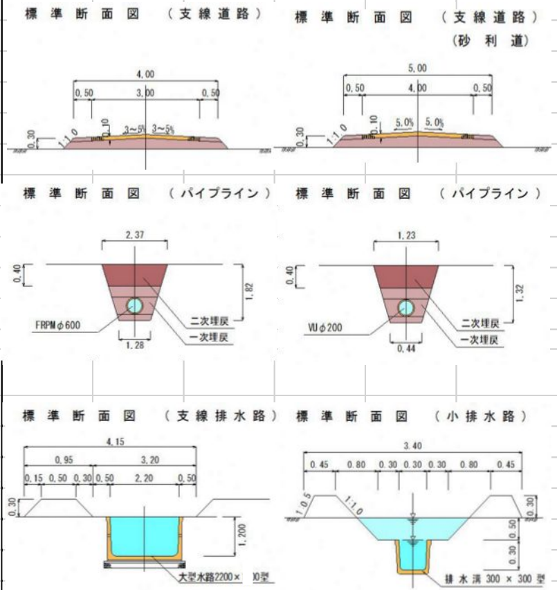
標準構造図
