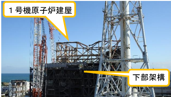
(写真1) 原子炉建屋西面
