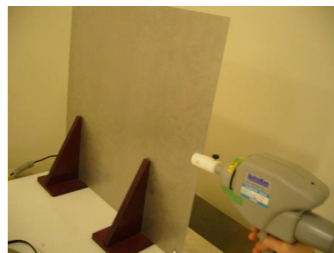
＜垂直結合板＞
