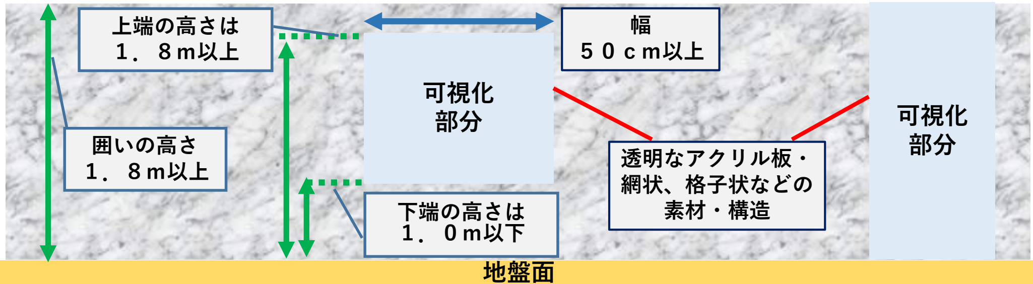
図 囲いの構造の例 (立面図)
