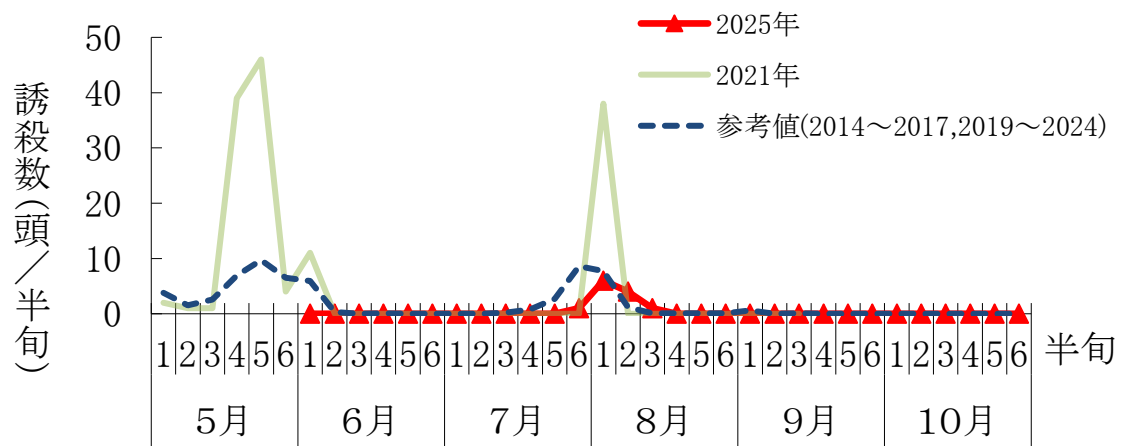
図1 フェロモントラップによるアメリカシロヒトリ誘殺状況 (郡山市日和田町)
