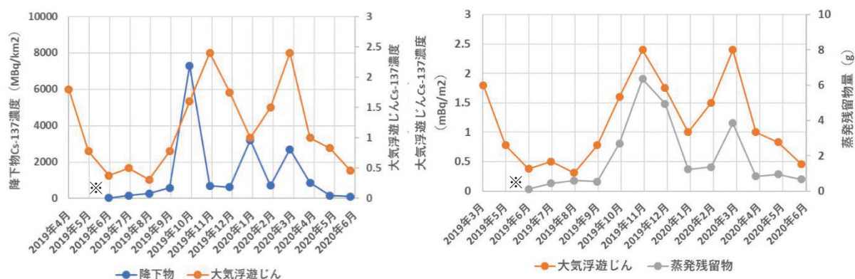
図4 降下物及び大気浮遊じん中のCs-137濃度測定結果（左） 大気浮遊じん中のCs-137放射能濃度と蒸発残留物量の関係（右）
