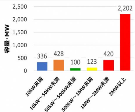
太陽光発電導入「容量」※2
