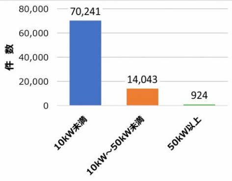
太陽光発電導入「件数」※2
