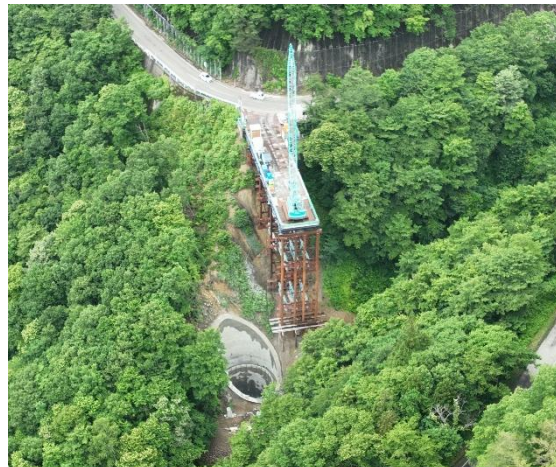
龍神橋 下部工(P1)
