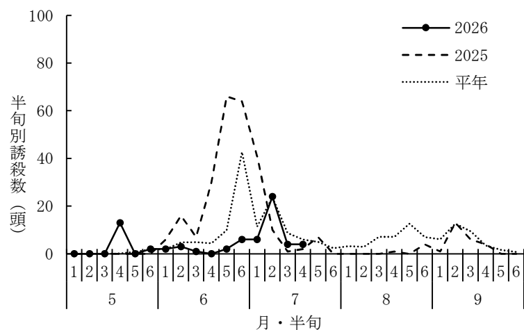
図7 予察灯によるアカスジカスミカメの誘殺状況
