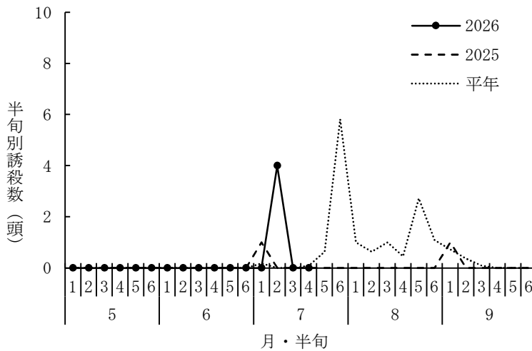
図2 予察灯によるセジロウンカの誘殺状況
