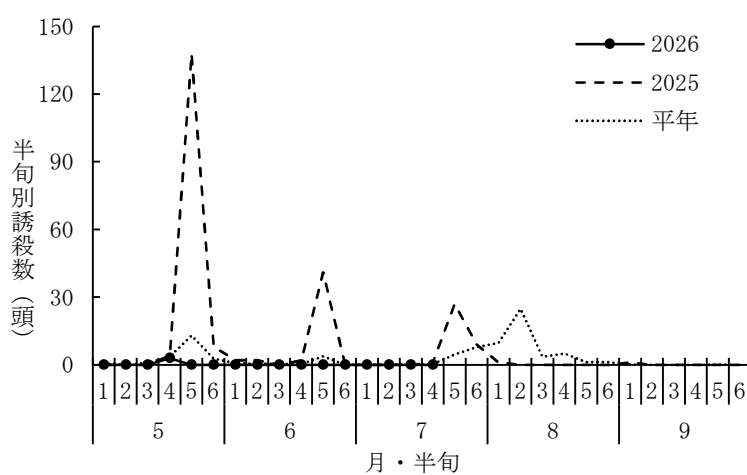
図6 予察灯によるイネミズゾウムシの誘殺状況
