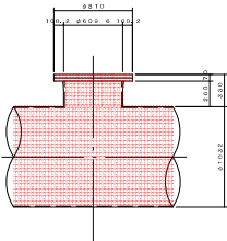
人 孔 管 S=1:30
