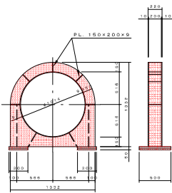
A 型 支 承 詳 細 S=1:30
