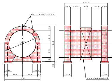
C 型 支 承 詳 細 S=1:30
