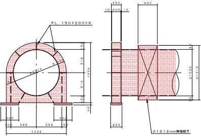
D 型 支 承 詳 細 S=1:30
