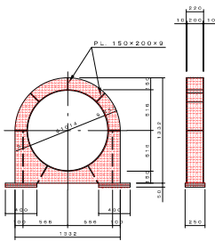
B 型 支 承 詳 細 S=1:30
