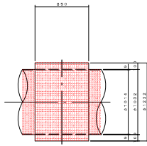
制 水 弁 S=1:30
