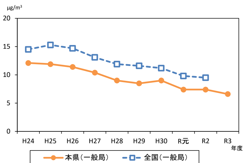
図2-1 本県及び全国の微小粒子物質（年平均値）の経年変化
