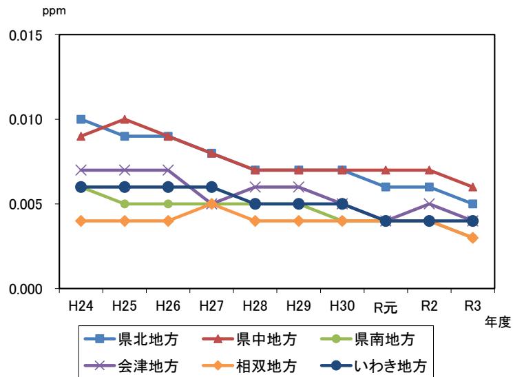
図 2-9 地方別の二酸化窒素濃度（年平均値）の推移
