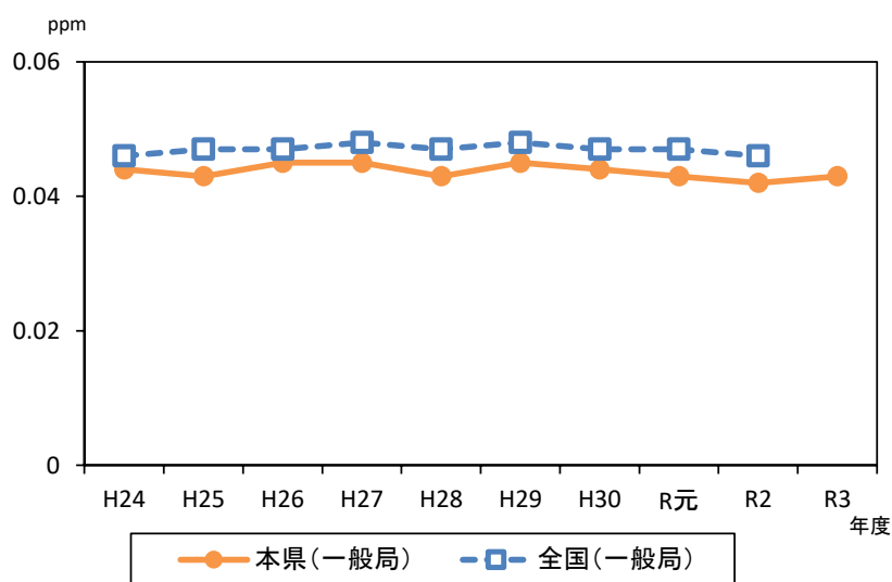
図2-4 本県及び全国の光化学オキシダント濃度の推移
