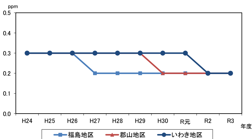
図 2-13 一酸化炭素濃度（年平均値）の経年変化
