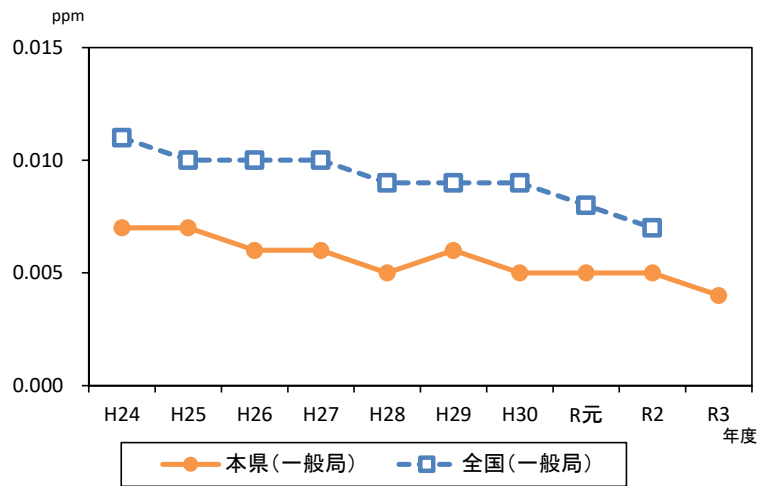
図 2-8 本県及び全国の二酸化窒素濃度（年平均値）の推移
