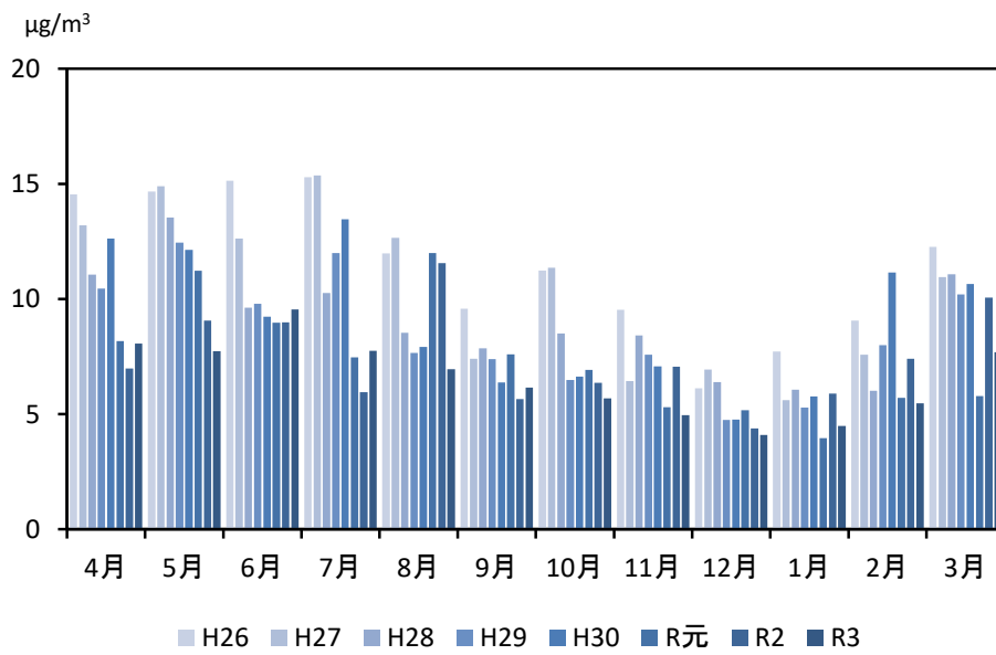
図 2 - 3 本県の微小粒子状物質（月平均値）の推移
