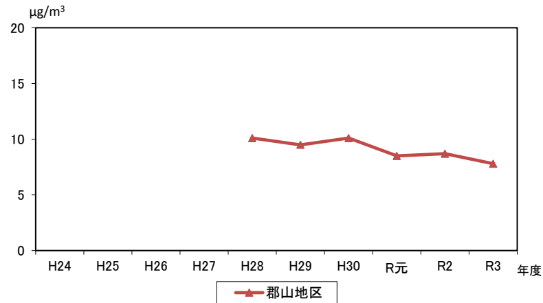
図 2-14 微小粒子状物質（年平均値）の経年変化
