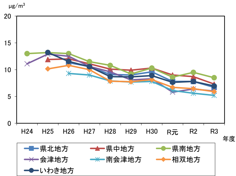
図 2 - 2 地方別の微小粒子状物質（年平均値）の経年変化
