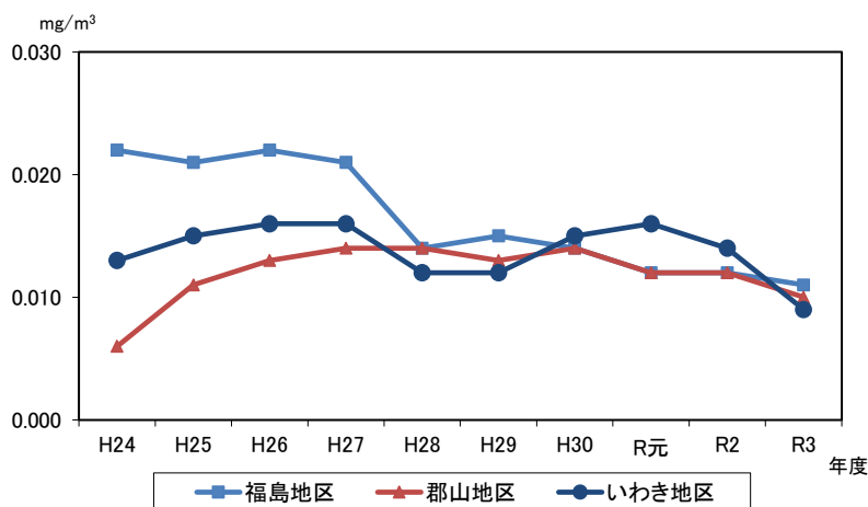
図2-17 浮遊粒子状物質（年平均値）の経年変化
