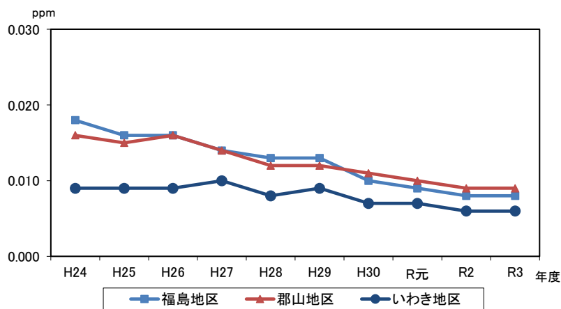
図 2-16 二酸化窒素（年平均値）の経年変化
