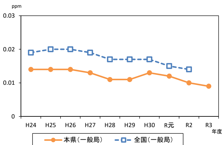
図 2-10 本県及び全国の浮遊粒子状物質（年平均値）の推移
