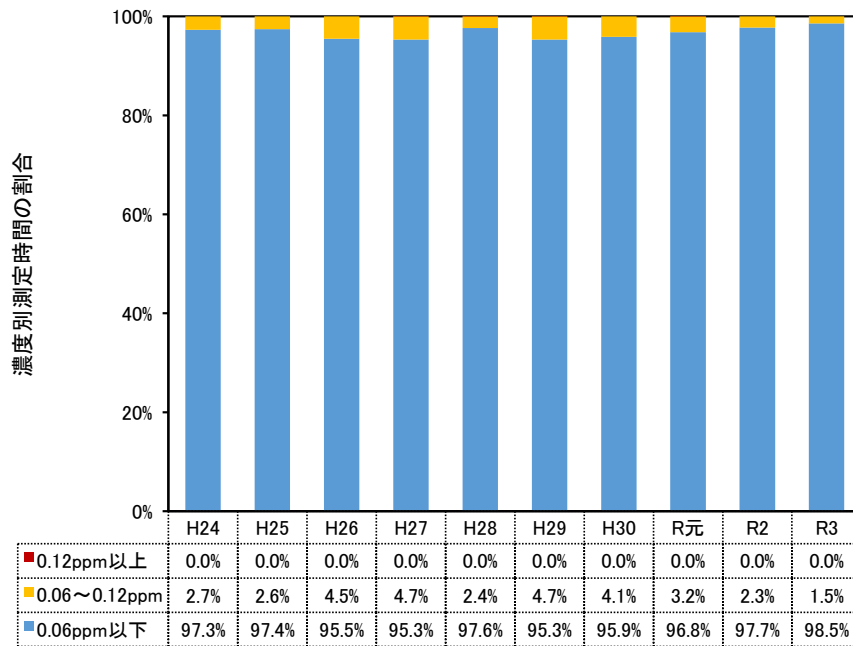
図 2-6 光化学オキシダント（昼間の 1 時間値）の濃度レベル別割合の推移
