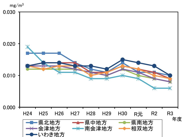
図 2-11 地方別の浮遊粒子状物質（年平均値）の推移
