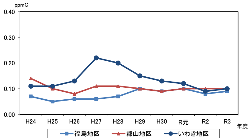
図 2-15 非メタン炭化水素（年平均値）の経年変化
