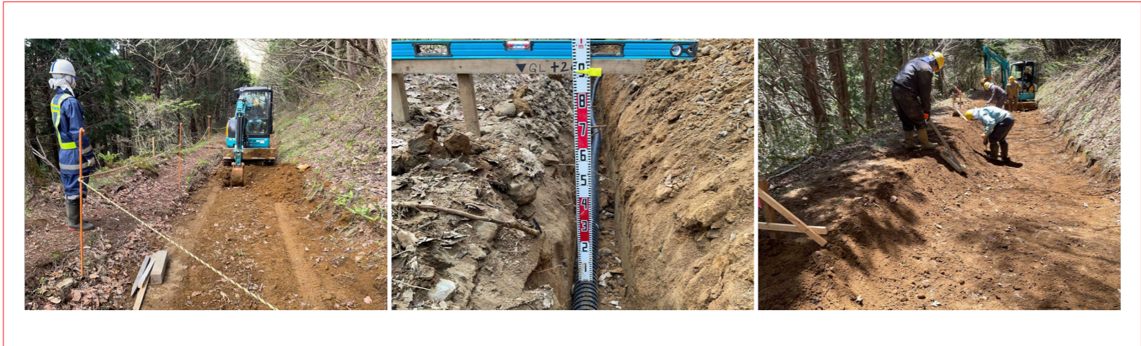
埋設配管敷設・接続ボックス設置作業写真 工事進捗91.1% (配管全長5420mの内4938m施工完了)
